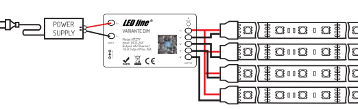
Abb.2 Installationschema
