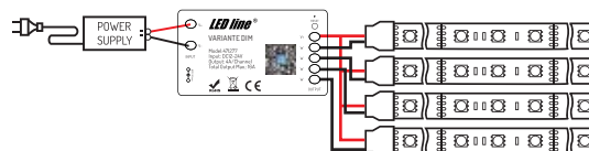
Rys.2 Schemat instalacji
