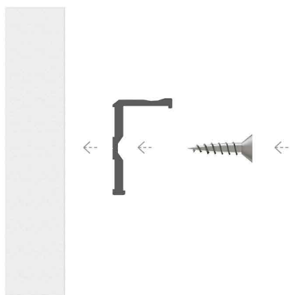
Instrukcja montażu profilu E za pomocą wkrętu montażowego
