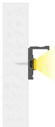
Efekt końcowy montażu profilu F za pomocą wkrętu montażowego
