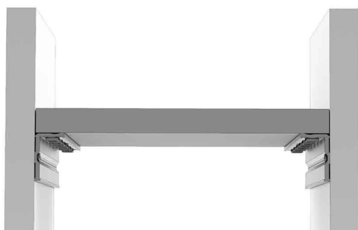
Schemat montażu profilu E pod półkami
